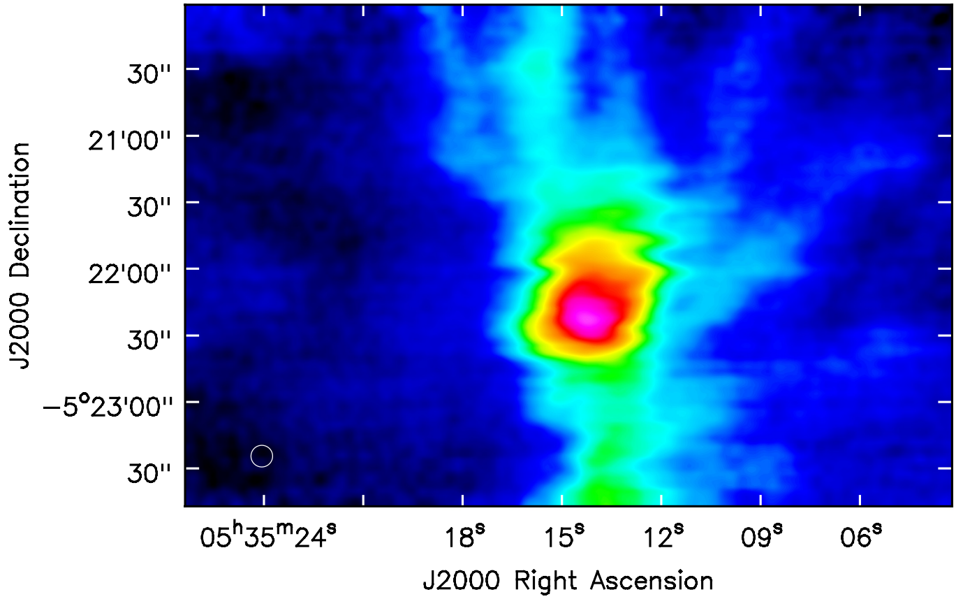
Argus: Orion HCN(1-0)
